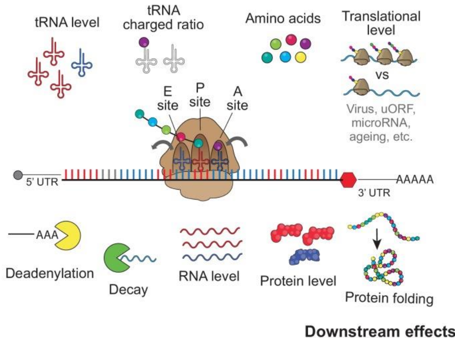
Fig. 2 il regolatore a monte e l'effetto a valle per l'ottimalità del codone Il livello di tRNA, il rapporto caricato con tRNA, l'amminoacido e il livello di traduzione potrebbero contribuire a regolare l'identità normativa e / o la forza di ciascun codone per influenzare l'espressione genica, influenzando la velocità di allungamento della traduzione. Gli effetti a valle del meccanismo meditato dal codone sono la deadenilazione dell'RNA, il decadimento dell'mRNA, il livello di mRNA, il livello di proteine e il ripiegamento delle proteine.
